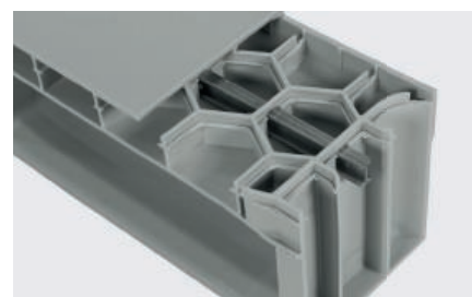
Met versterkingsprofielen
