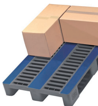
CR1 met blauwe antislipstroken
