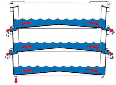
Gewelfde bodem met afwateringsgaten in de hoeken
